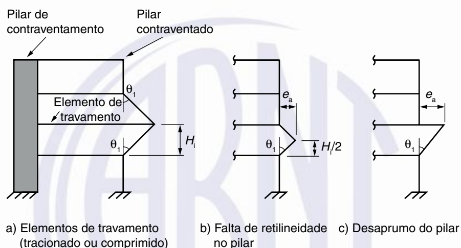
Figura 11.2 – Imperfeições geométricas locais
