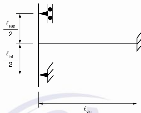
Figura 14.8 – Aproximação em apoios extremos
