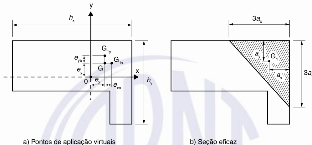
Figura 24.2 – Seção flexo-comprimida
