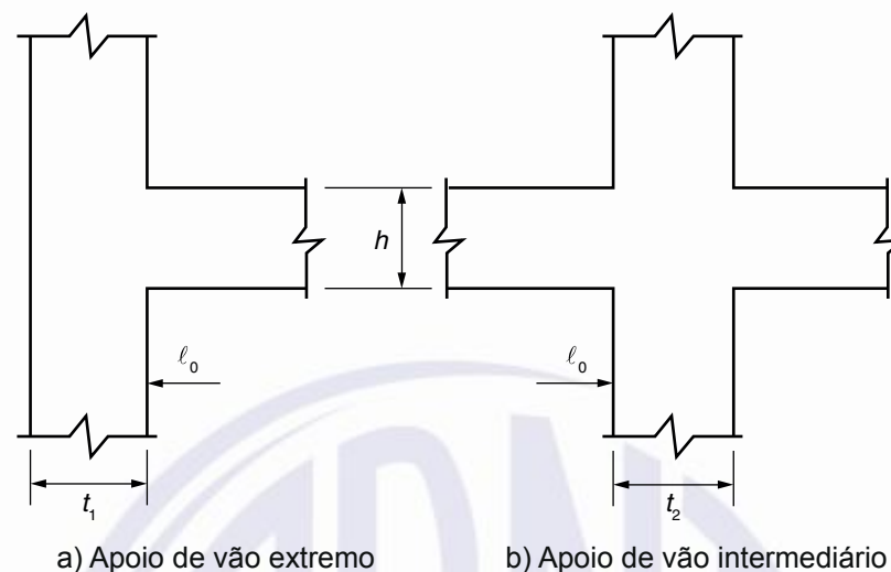
Figura 14.5 – Vão efetivo
