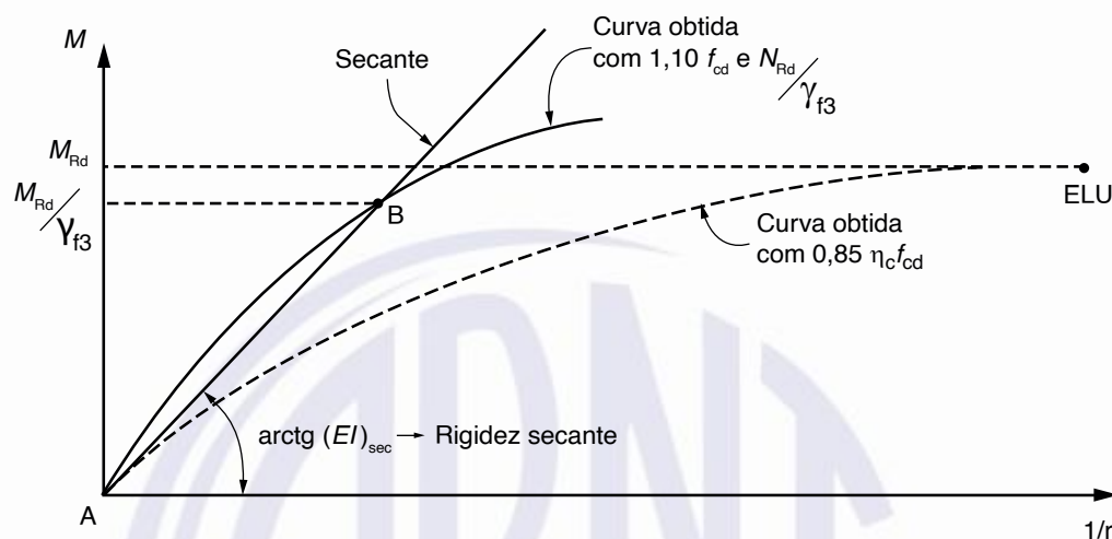
Figura 15.1 – Relação momento-curvatura
