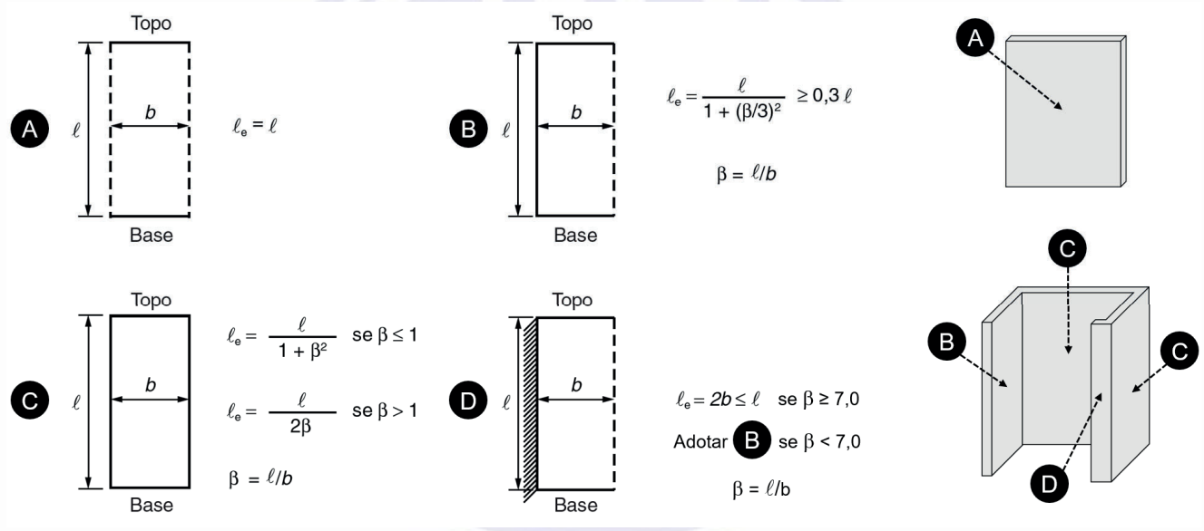
Figura 15.4 – Comprimento equivalente \ell_e
