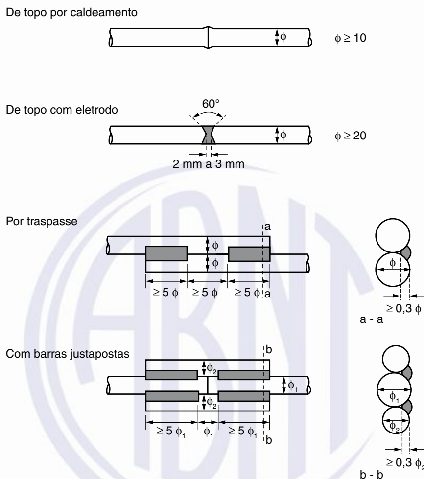
Figura 9.6 – Emendas por solda
