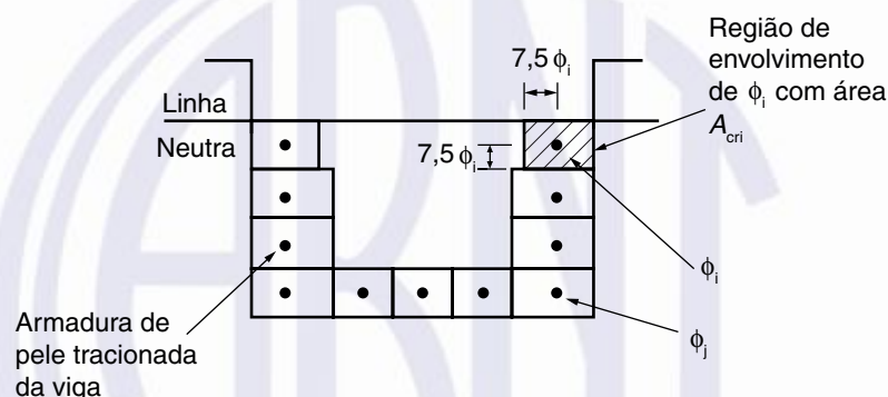
Figura 17.4 – Concreto de envolvimento da armadura
