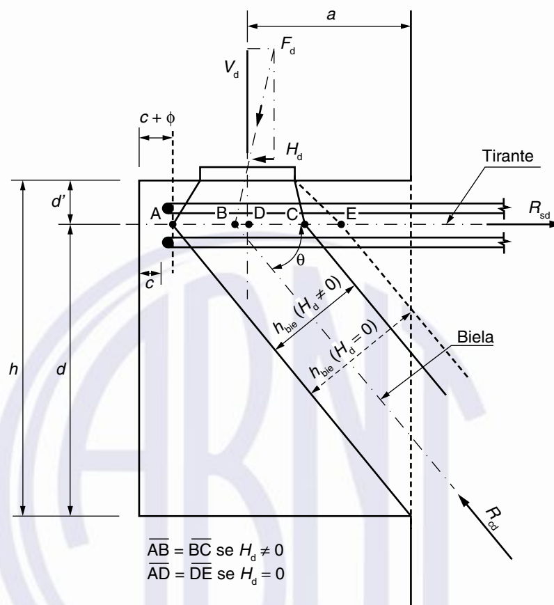
Figura 22.4 – Modelo biela-tirante para consolo curto
