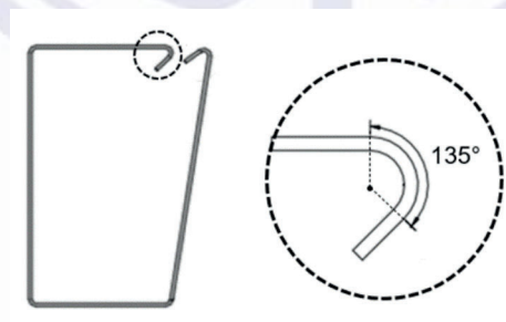
Figura 9.2 – Estribo com gancho em 135°
