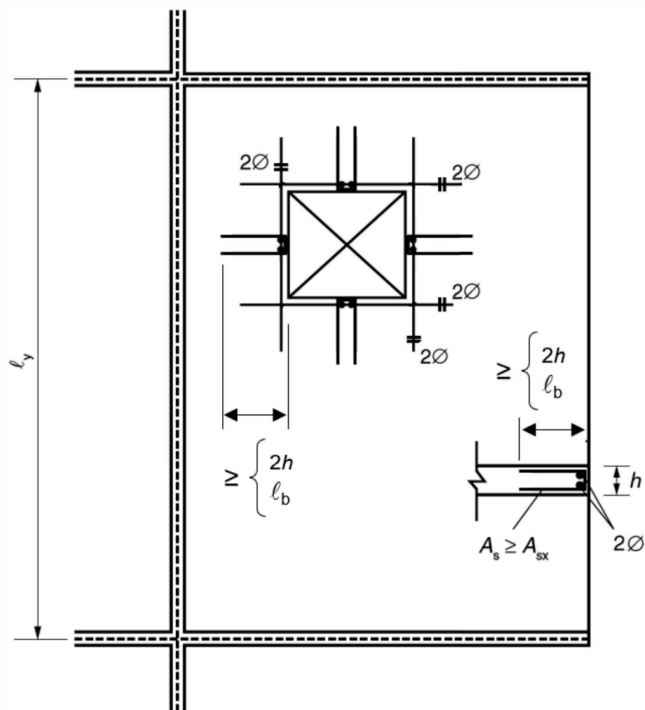
Figura 20.1 – Bordas livres e aberturas das lajes maciças
